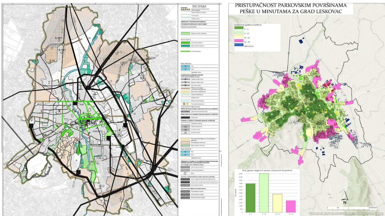
Слика бр. 5 (лево). Приступачност зеленим површинама у Лесковцу (Извор: Ивана Момић, софтвер ArcGIS Pro); Слика бр. 6. (десно). Систем зелених површина града Лесковца (Извор: Генерални урбанистички план Лесковца);
