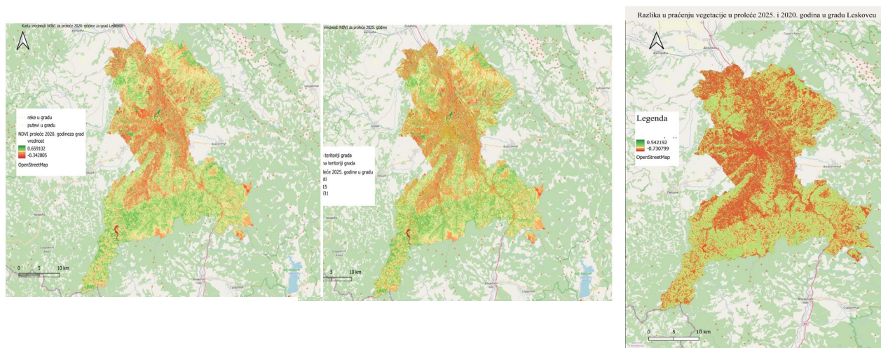
Слика 10: Карта вредности NDVI за пролеће 2020 и 2025. године у граду Лесковцу и \Delta \text{NDVI} (Извор: Истраживања – примена Сентинел-2 података у анализи зелених површина у урбаним срединама – студија случаја града Лесковца)
