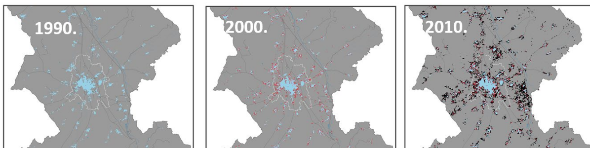
Слика бр. 4: Изграђено подручје унутар ГУП Лесковац и околини 1990 (плаво), 2000. (црвено) и 2020. године (црно) (Извор: GHSL_BUILD S, built-up area у резолуцији од 100 m 2 за 1990, 2000. и 2020. годину)
